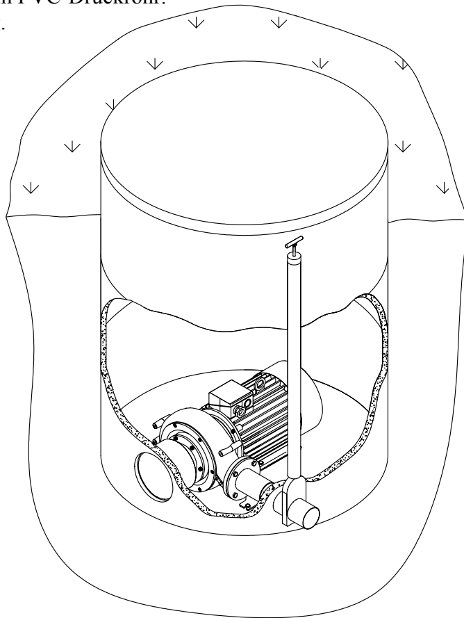
Prinzipskizze 3740698
